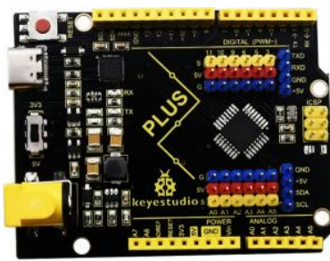
Плата управления
