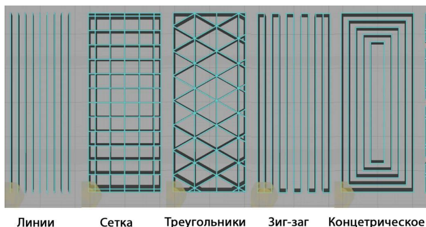
Рис.2. Виды поддержек
