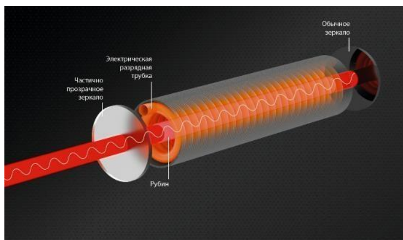
Рисунок 1 - Принцип действия лазера
