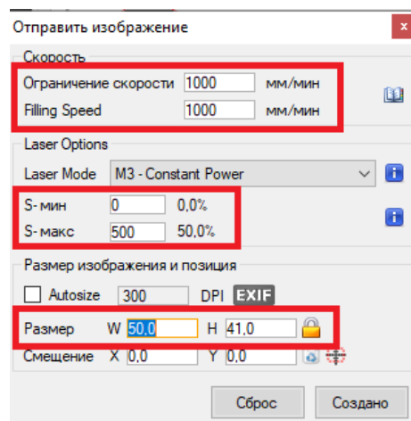
Рисунок 8 - Параметры для гравировки
