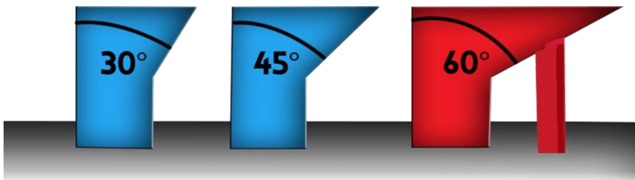
Рис.5. Модель с поддержками и без.
