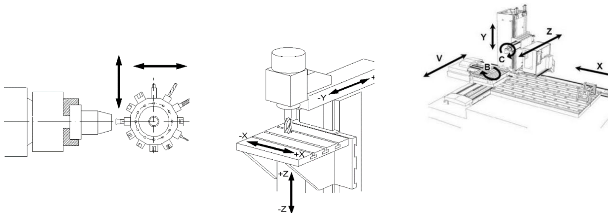
2 - сурет-а) токарлық станок (2 ось), б) фрезерлік станок (3 ось), в) әмбебап станок (көп ось)
