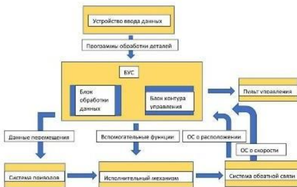
41-сурет-СББ машинасының құрылымдық схемасы
