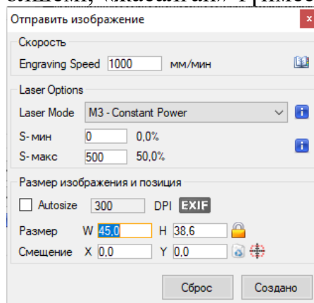
89-сурет. Гравюра машинасының параметрлерінің
