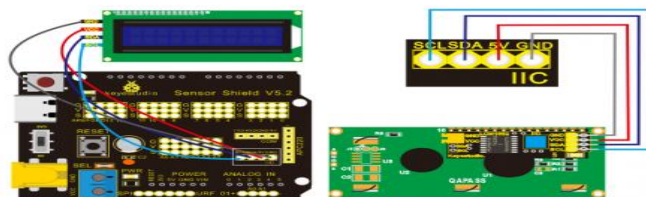
34-сурет - Контроллерді контроллерге қосу.
