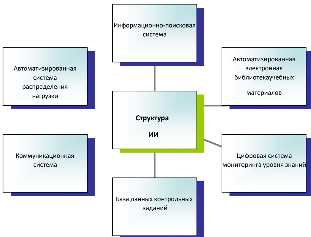
Рисунок 3 – Структура ИИ
