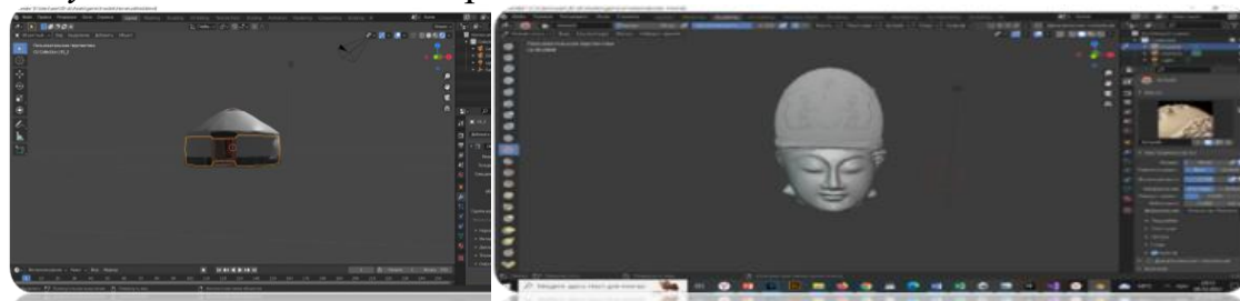
Рисунок 2. «Написание скрипта»
