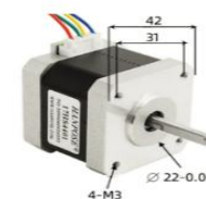
Stepper Motor 17HS4401
